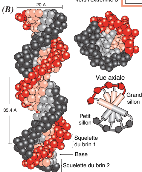
Modèle moléculaire
