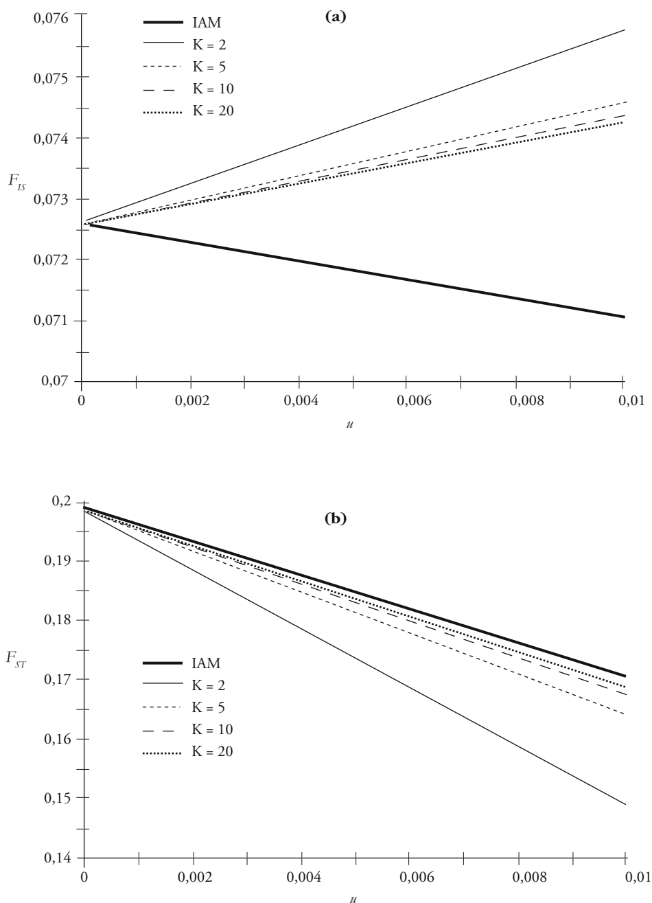
Figure 9 Illustration de l'influence du nombre d'allèles possibles ( K ) sur les valeurs attendues des F statistiques de Wright, pour différents taux de mutation ( u ). Les valeurs sont obtenues pour un modèle en îles infini avec N = 20 individus par sous-population, un taux d'autofécondation de s = 0,2 et un taux de migration de m = 0,05 (IAM = nombre infini d'allèles).
