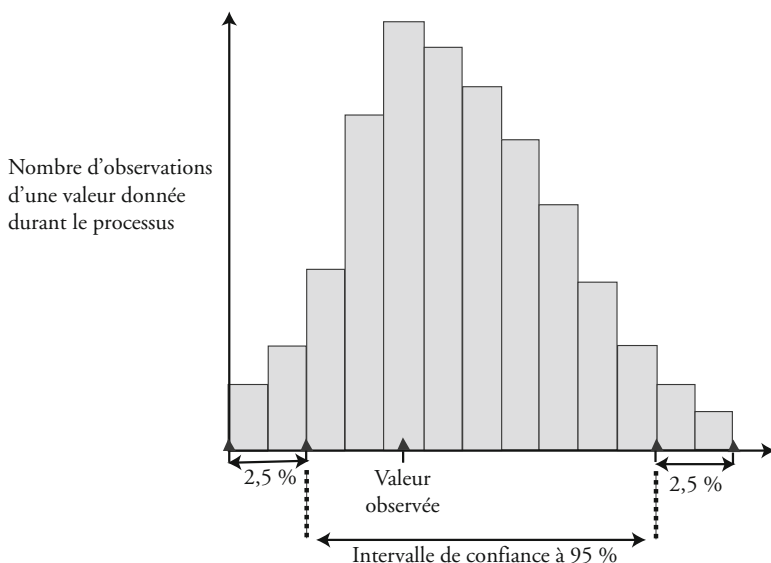
Figure 10 Représentation graphique de l'obtention de l'intervalle de confiance à 95 % d'une mesure à partir de la technique du bootstrap.
